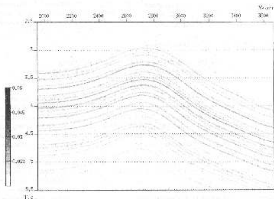
Рис. 4. Синтетический временной разрез по сейсмическому профилю без учета изменения давления.
