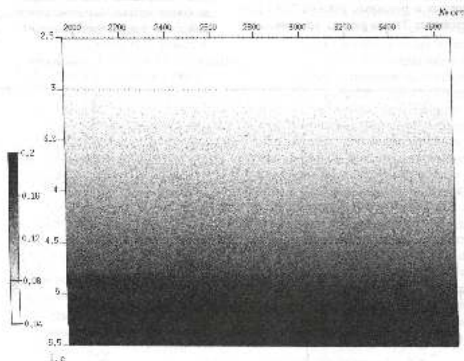
Рис. 2. Модель распределения геостатического давления по сейсмическому профилю
