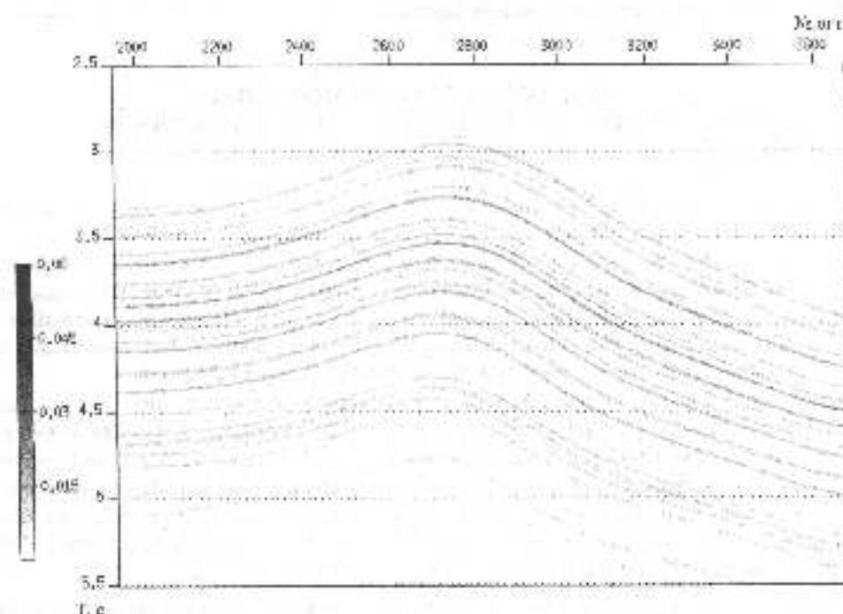
Рис. 5. Синтетический временной разрез по сейсмическому профилю после коррекции пластических скоростей с учетом изменения давления
