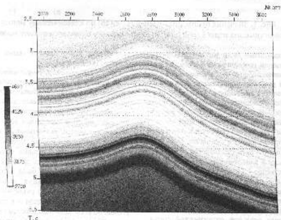
Рис. 3. Тонкослойная модель распределения пластовых скоростей по сейсмическому профилю
